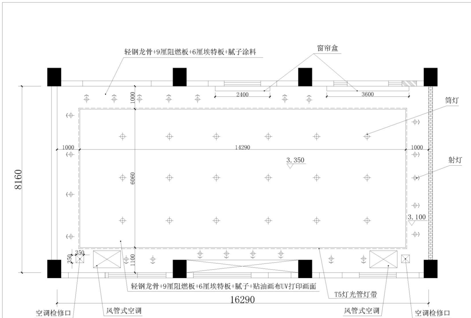
无人机教室天花布置图
