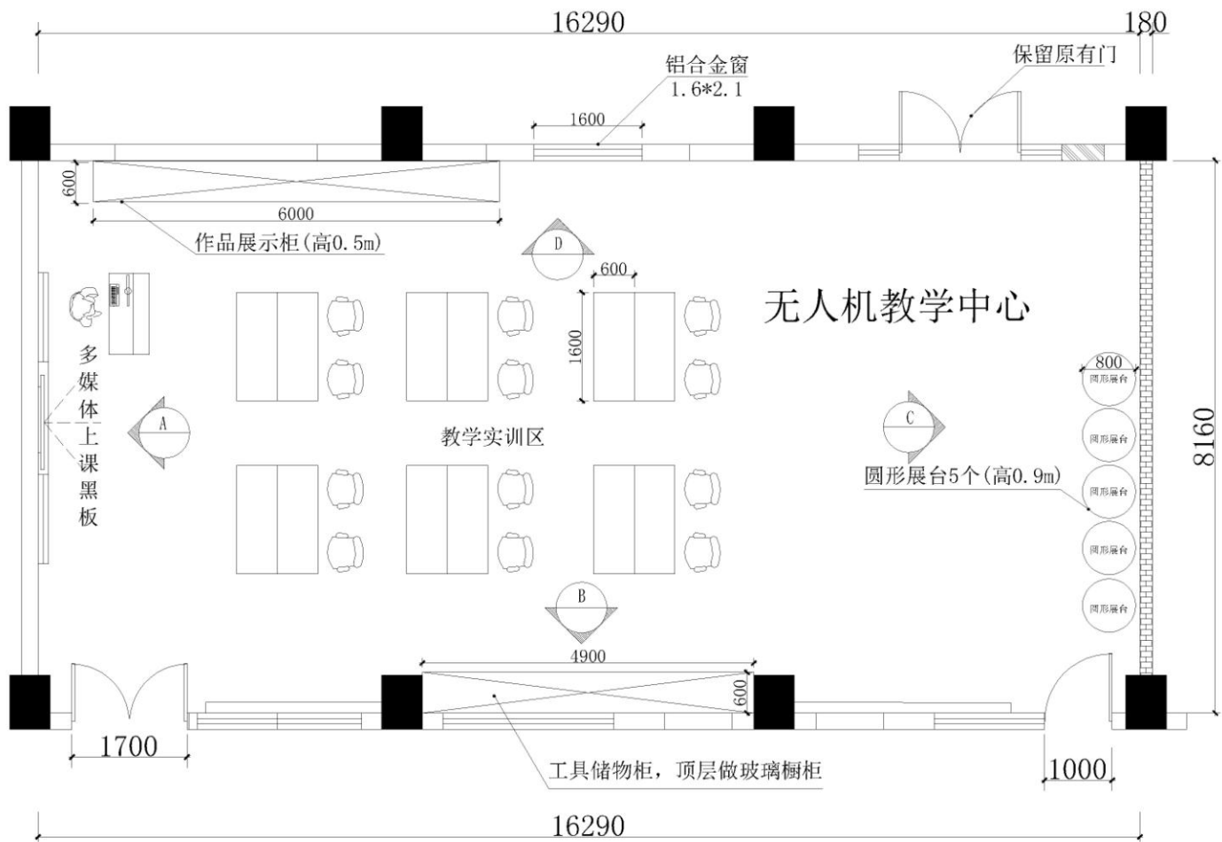
无人机教室平面布置图
