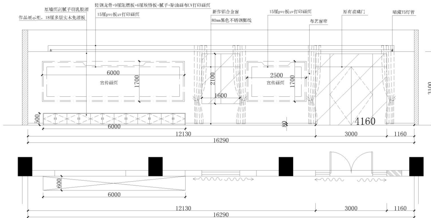
无人机教室D立面图
