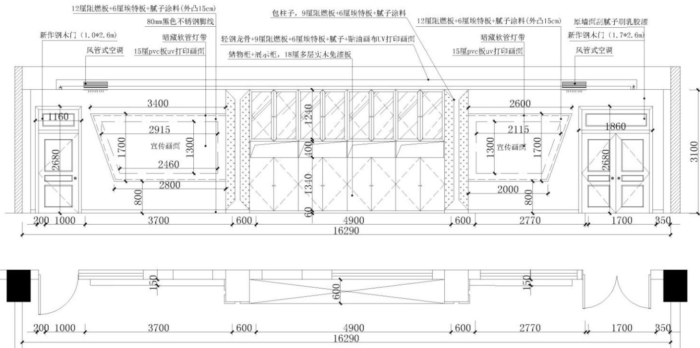
无人机教室B立面图
