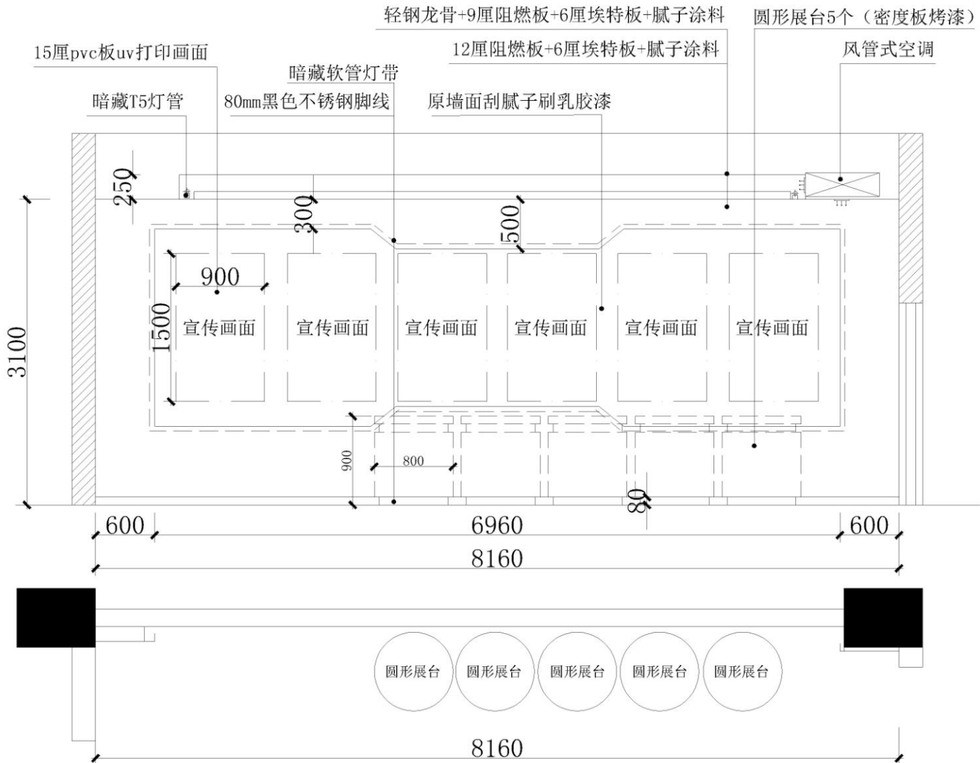
无人机教室C立面图
